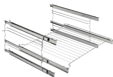
Afbeelding: PZ1503 Telescopische geleiding 3-voudig voor JUNO
